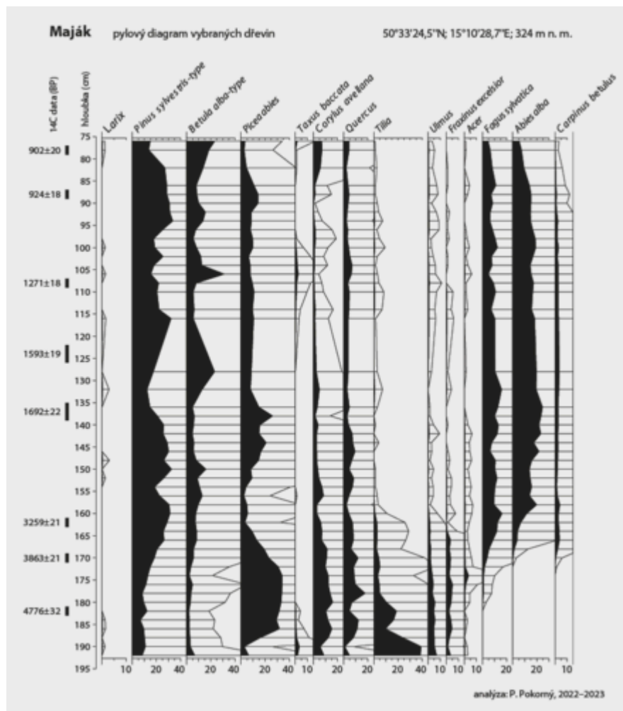
Zjednodušený pylový diagram z vrtu rašelinou v lokalitě Maják v Českém ráji. Autor Petr Pokorný
